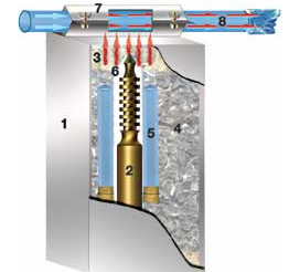
Dynamiseur Spécial pour bâtiments - conduites de 2.5 à 3.2 cm
